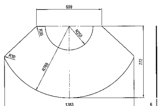
Saison-Funkenschutzplatte 23/2290.2909
