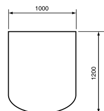
Korbbogen- Funkenschutzplatte
