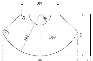
Saison-Funkenschutzplatte 23/2290.2911
