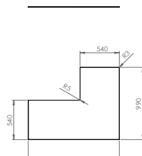
Saison-Funkenschutzplatte 41/6361.2901
