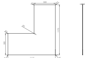
Saison-Funkenschutzplatte 41/6051.2901
