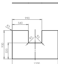
Saison-Funkenschutzplatte 41/6461.2901
