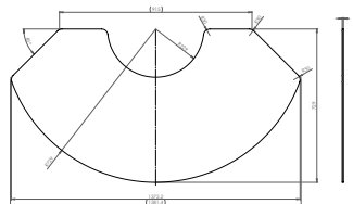
Saison-Funkenschutzplatte 23/2290.2912
