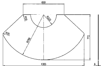
Saison-Funkenschutzplatte 23/2290.2910
