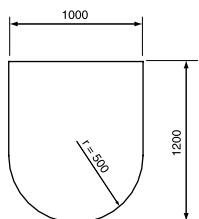
Rundbogen- Funkenschutzplatte
