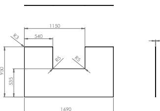
Saison-Funkenschutzplatte 41/6161.2901
